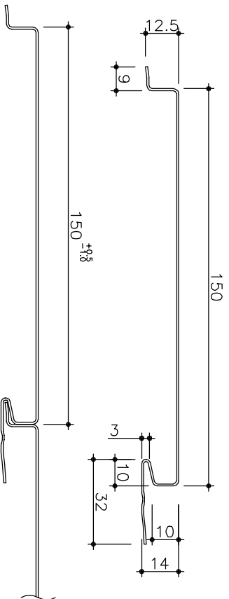
AF155タイプ AF150F型 働き巾150 +0.5 -1.0 t=0.8 (目地なしタイプ)
