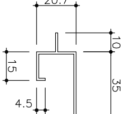
NC-101S 底目地廻り縁
