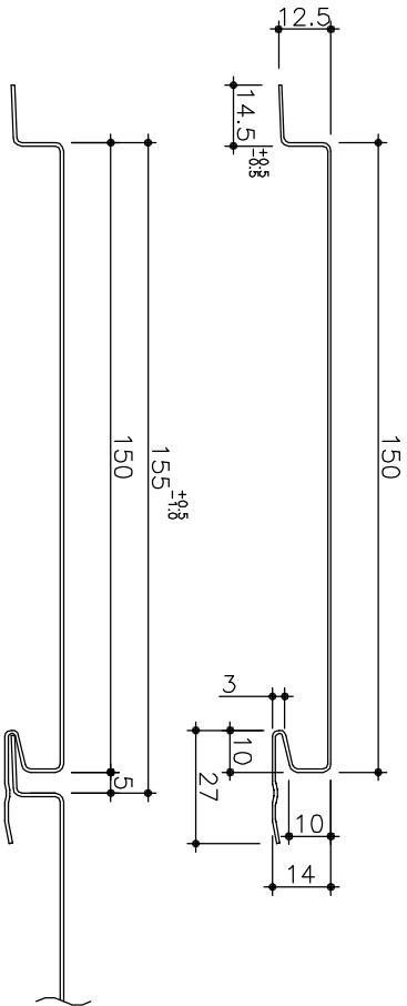
AF155タイプ AF155F型 働き巾155 +0.5 -1.0 t=0.8 (目地ありタイプ)
