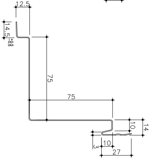
NC-304 入隅 (目地あり用)
