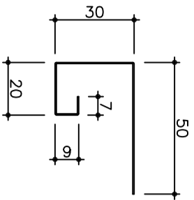
廻り縁 K-101 2m
