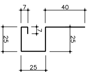
腰水切り C-250 2m
