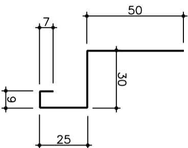
水切 K-202 2m
