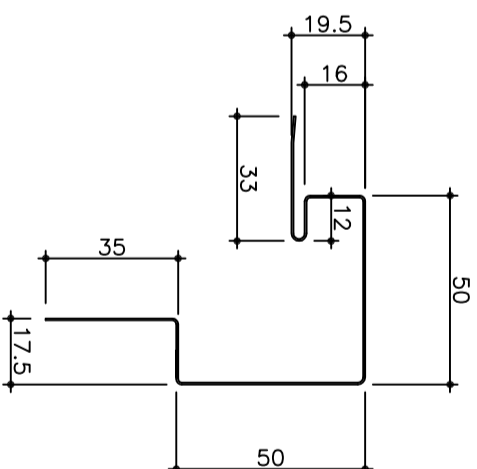
出隅 (K-303)
