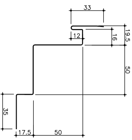
入隅 (K-304)
