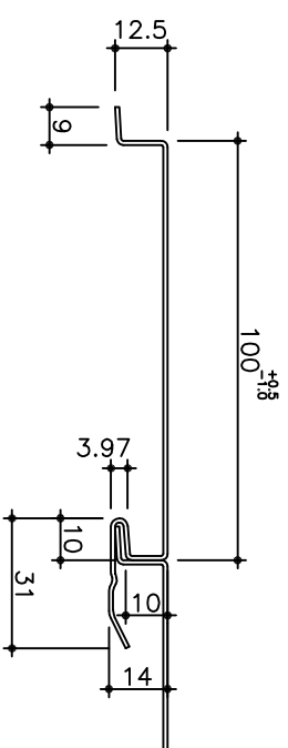
AF105タイプ AF100型 動き巾100 +0.8 t=1.0 (目地なしタイプ)
