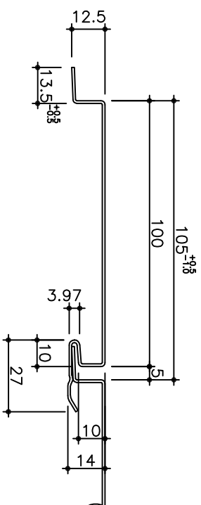
AF105タイプ AF105型 動き巾105 +0.8 t=1.0 (目地ありタイプ)
