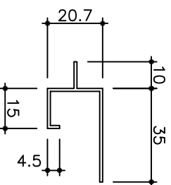
NC-101S 底目地廻り縁
