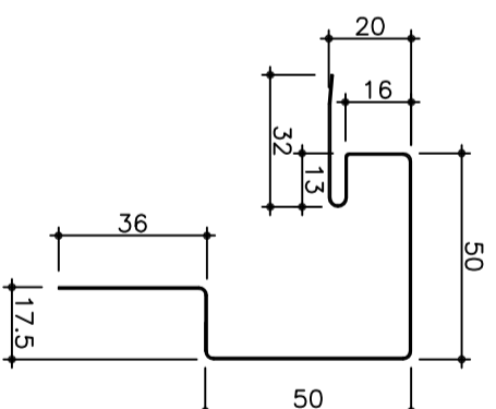
出隅 (SK-303) (0.4t)
