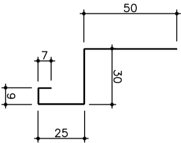
水切 SK-202 2m (0.4t)
