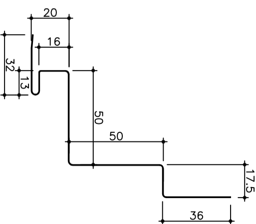
入隅 (SK-304) (0.4t)
